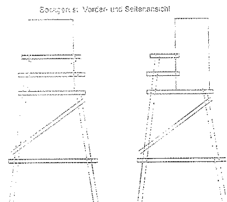
So sieht der Hochsitz, den die Schüler der LFS Stainz bauen werden, am Papier aus.
